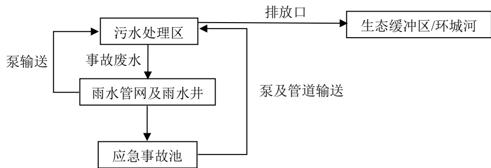
图 4-2 事故废水收集系统图
