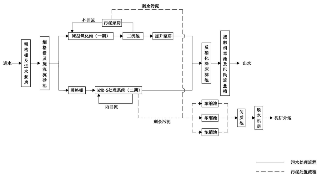
图 2-5 张家港城北污水处理有限公司污水处理工艺流程图
